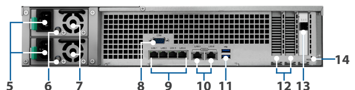
Задняя панель
