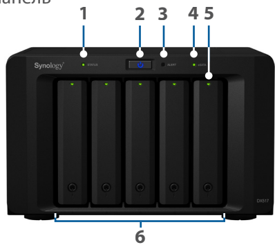
Передняя панель
